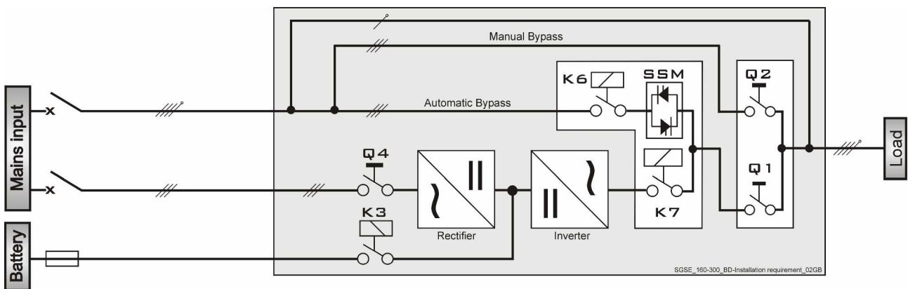
Одиночный ИБП с отдельными входами выпрямителя и байпаса
