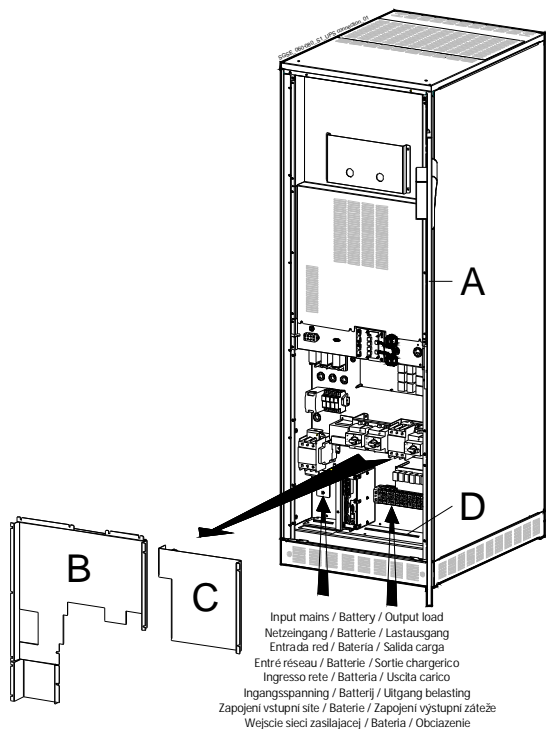
Рис. 5.6-1 SG-CE Series 60 – 80 кВА PurePulse® Доступ к силовым шинам
