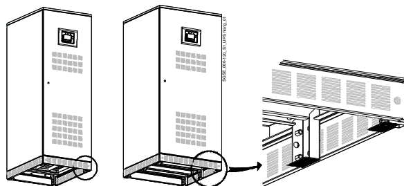
Рис. 5.4.1-4 Крепление шкафа ИБП к полу
