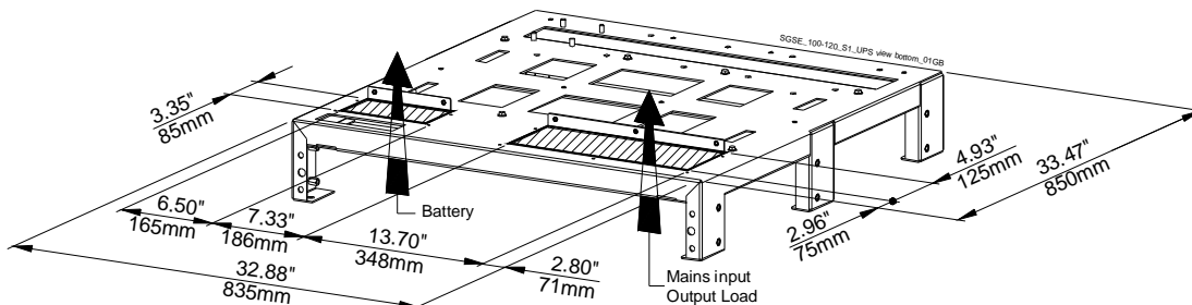
Рис. 5.4.1-3 SG-CE Series 100 – 120 кВА PurePulse® - Отверстия в нижней части шкафа ИБП для ввода силовых кабелей
