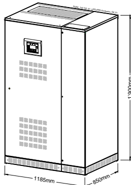
SG-CE Series 100 – 120кВА PurePulse® с фильтром EMC (опция)
