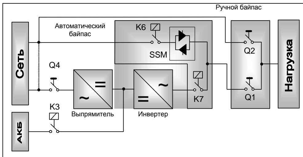
Рис. 4.1-1 Блок-схема ИБП
