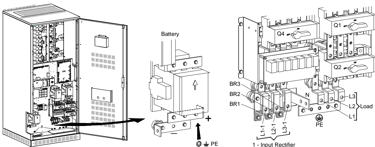
Рис. 5.6.3-1 SG-CE Series 100 – 120 кВА PurePulse® - Подключение силовых кабелей, общий вход выпрямителя и байпаса
