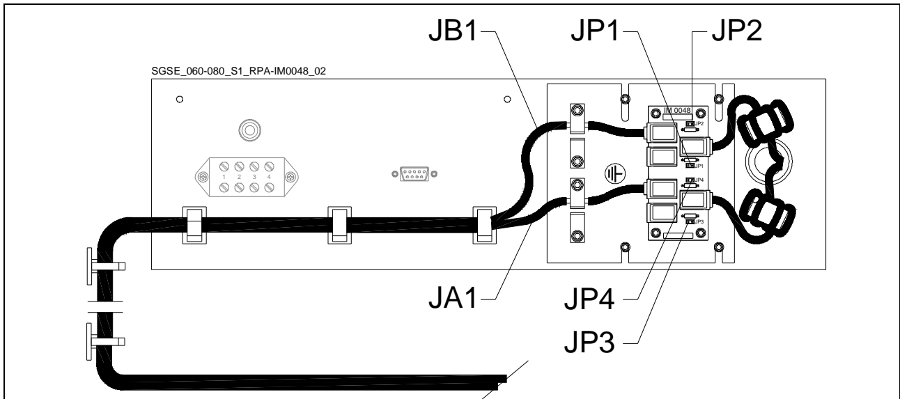
Рис. 5.9.2-2 Подключение информационного кабеля на первом и последнем ИБП
