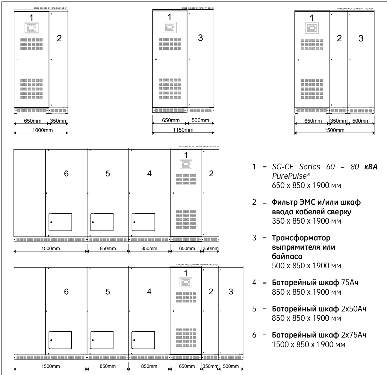
Вес ИБП SG-CE Series 60 – 80 кВА PurePulse® и опций
