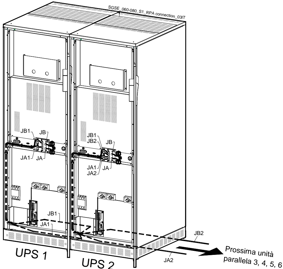
Рис. 5.9.3-3 Прокладка кабелей шины управления
