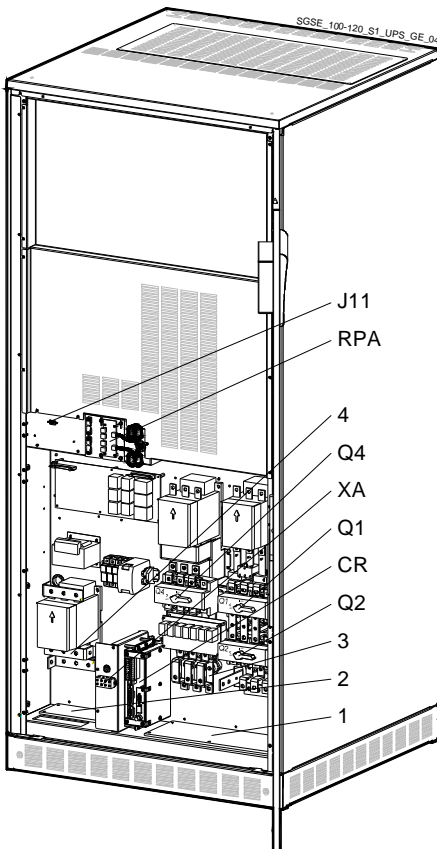
Рис. 2.3-3 Общий вид со снятыми защитными панелями
