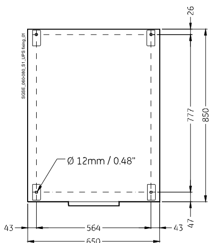
Рис. 5.4.1-5 SG-CE Series 60–80 кВА PurePulse® Точки крепления ИБП к полу
