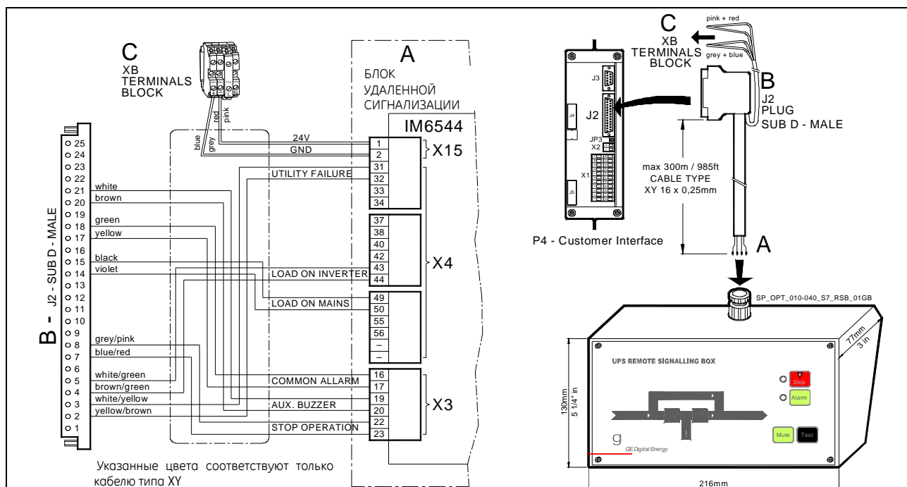
Рис. 10.6.3-1 Подключение удаленного сигнального устройства
