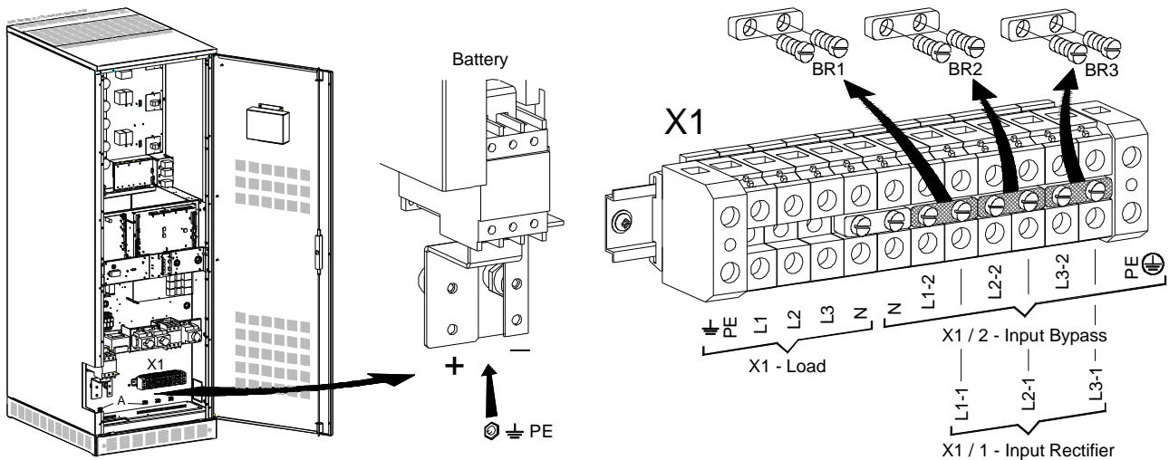
Рис. 5.6.2-1 SG-CE Series 60 – 80 кВА PurePulse® - Подключение силовых кабелей, отдельные входы выпрямителя и байпаса
