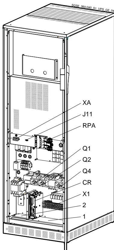
Рис. 2.1-3 Общий вид со снятыми защитными панелями
