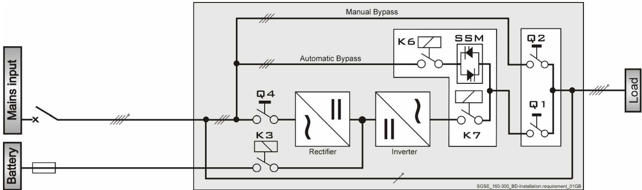
Одиночный ИБП с общим входом выпрямителя и байпаса
