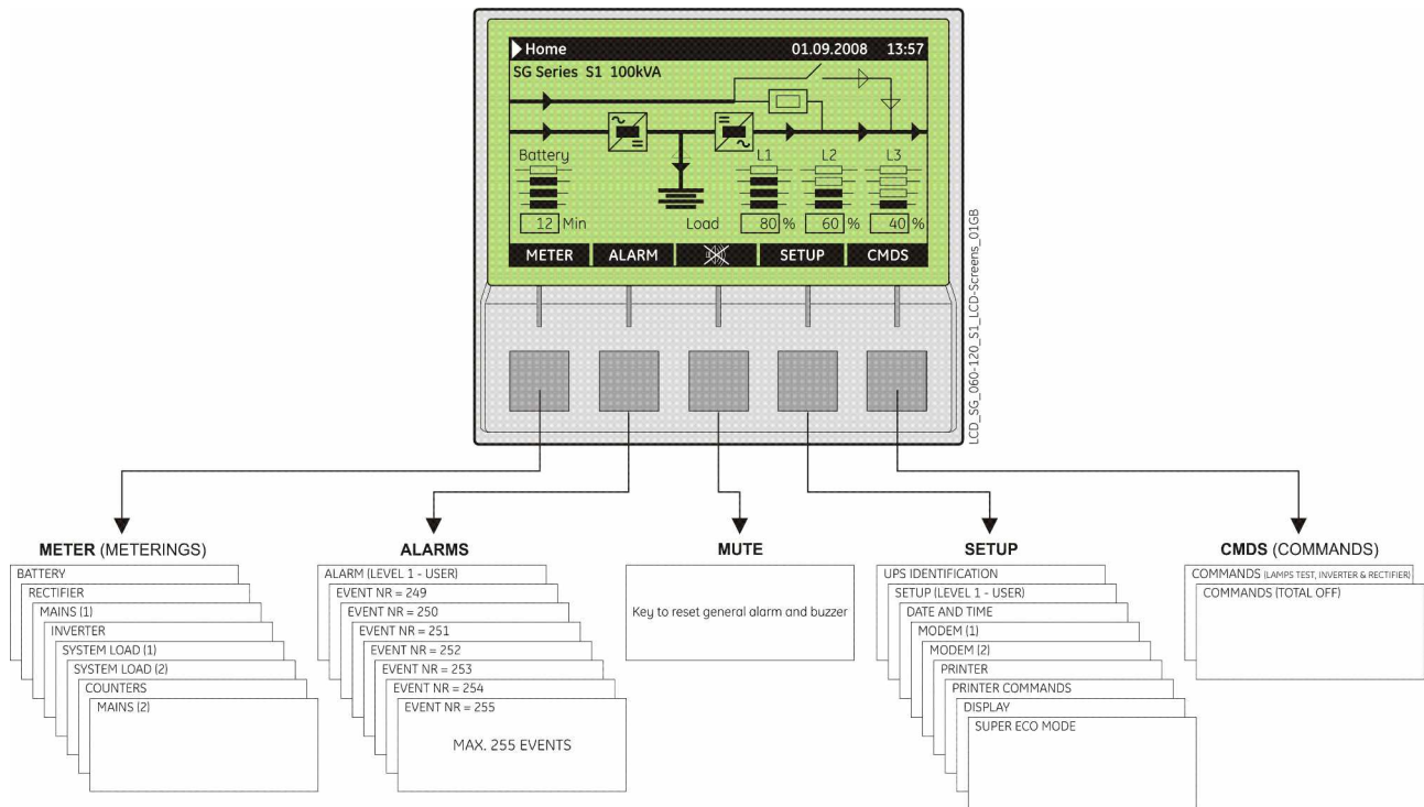
Рис. 7.1-1 ЖК-дисплей
