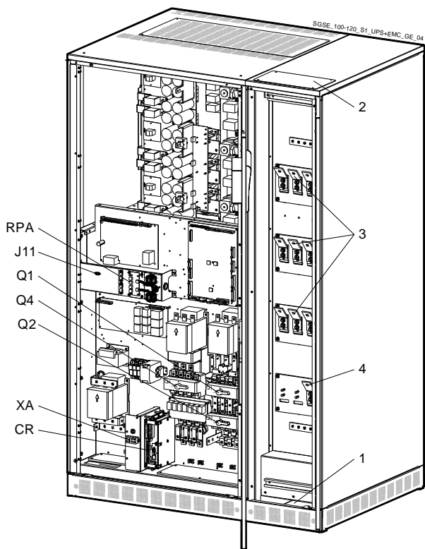
Рис. 2.4-3 Общий вид со снятыми защитными панелями
