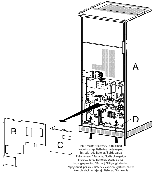
Рис. 5.6-2 SG-CE Series 100 – 120 кВА PurePulse® Доступ к силовым шинам
