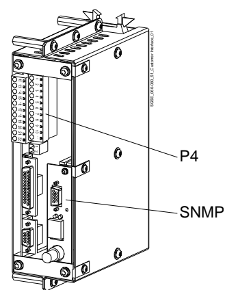
Рис. 2.1-5 Блок интерфейсов
