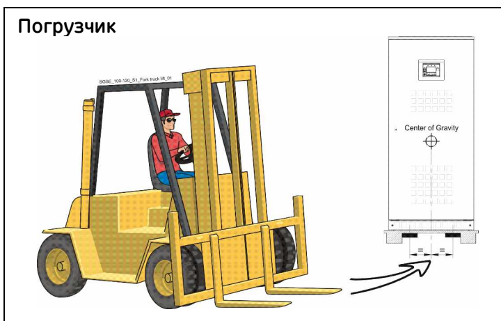
Рис. 5.1-1 Транспортировка нераспакованного ИБП погрузчиком
