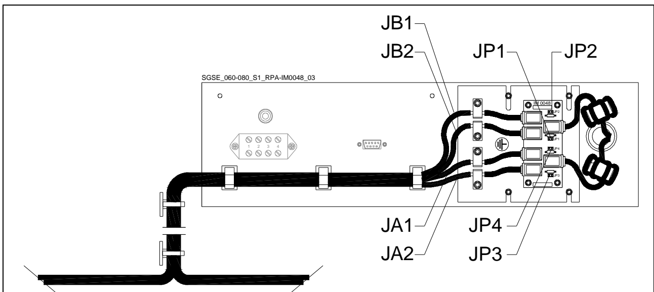
Рис. 5.9.2-3 Подключение информационного кабеля на промежуточных ИБП
