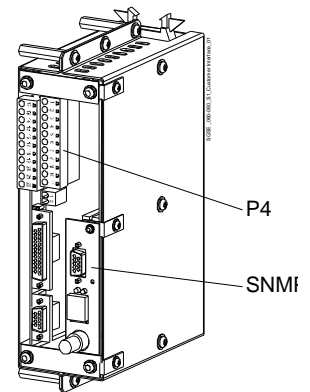
Рис. 2.3-5 Блок интерфейсов
