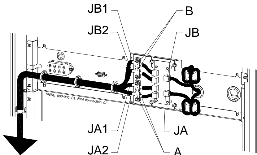
Рис. 5.9.3-2 Вид спереди на блок электроники промежуточных ИБП
