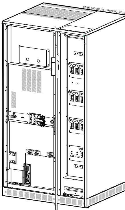
Рис. 2.2-2 Общий вид с открытой дверью
