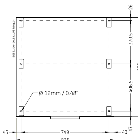
Рис. 5.4.1-4 Крепление шкафа ИБП к полу
