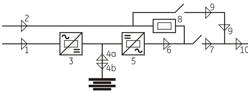
Рис. 7.1-2 Индикаторы на мнемосхеме
