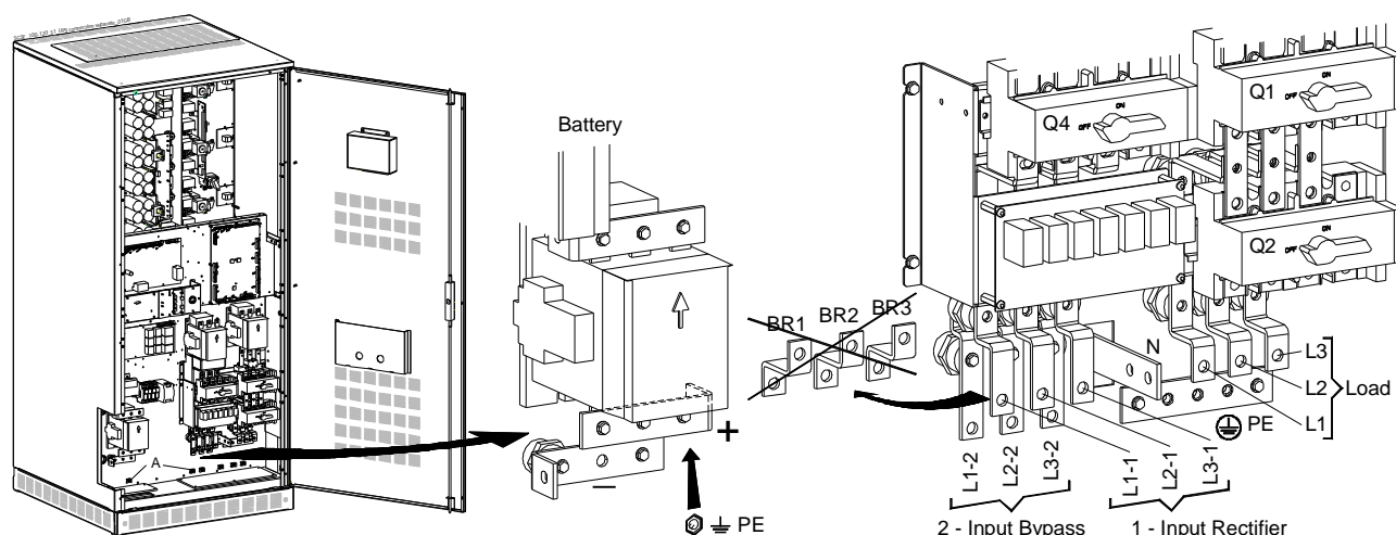
Рис. 5.6.4-1 SG-CE Series 100 – 120 кВА PurePulse® - Подключение силовых кабелей, раздельные входы выпрямителя и байпаса
