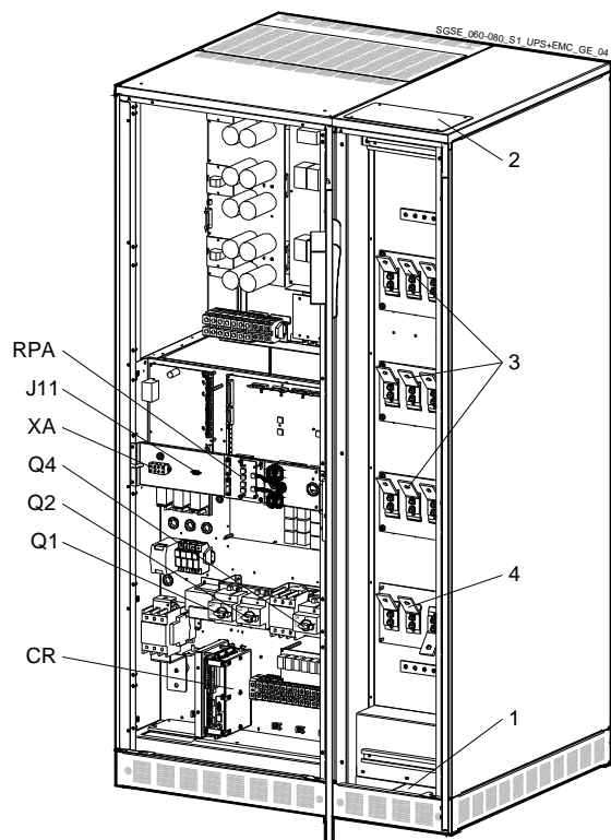
Рис. 2.2-3 Общий вид со снятыми защитными панелями
