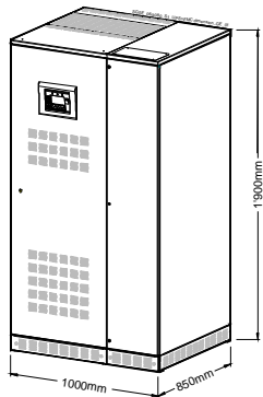
SG-CE Series 100 – 120кВА PurePulse® с фильтром EMC (опция)
