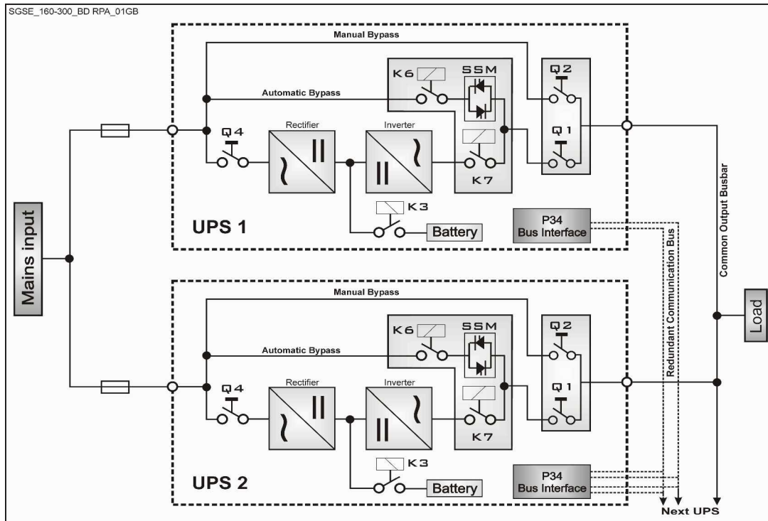
Рис. 4.3.1-1 ИБП - схема параллельной системы
