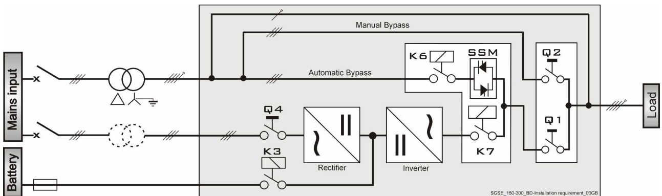
Одиночный ИБП с отдельными входами выпрямителя и байпаса и гальванической развязкой
