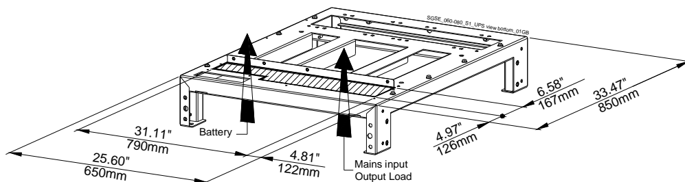
Рис. 5.4.1-2 SG-CE Series 60 – 80 кВА PurePulse® - Отверстия в нижней части шкафа ИБП для ввода силовых кабелей
