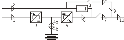
Мнемосхема на первом ИБП
