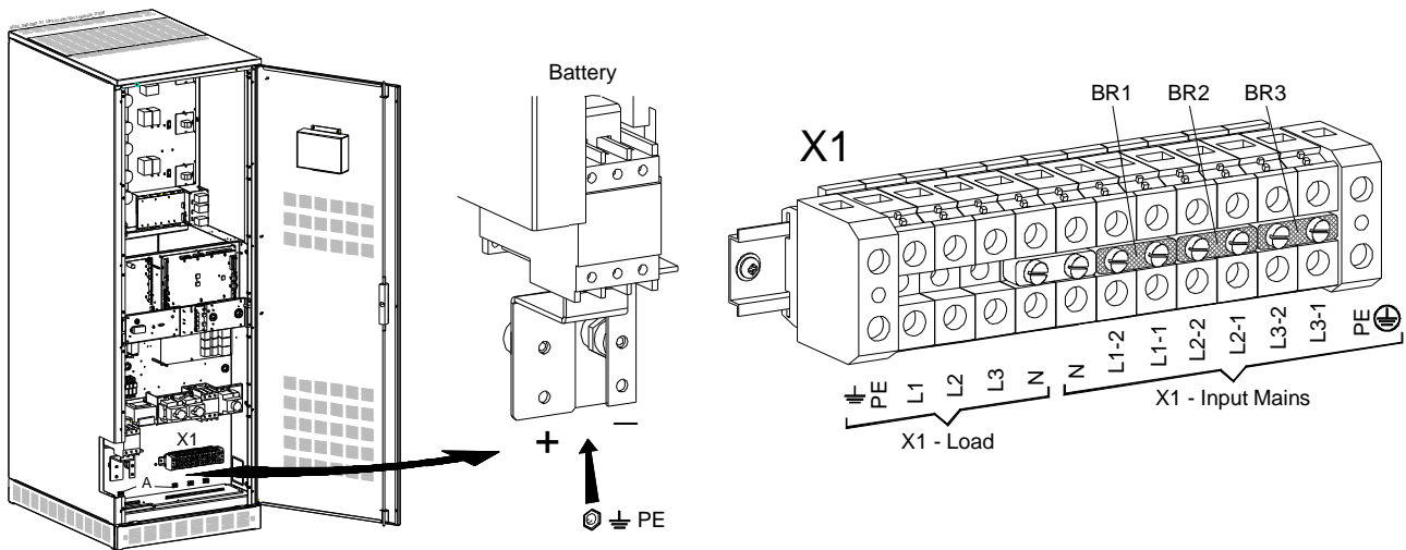
Рис. 5.6.1-1 SG-CE Series 60 – 80 кВА PurePulse® - Подключение силовых кабелей, общий вход выпрямителя и байпаса
