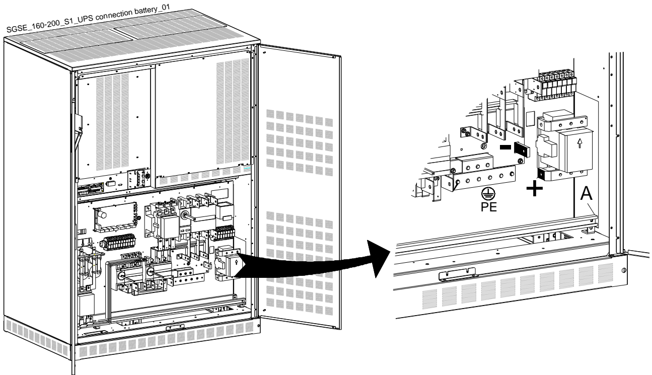
Рис. 5.8.5-1 Подключение батареи
