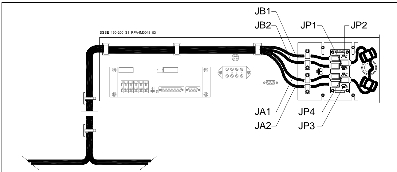
Рис. 5.9.2-3 Подключение информационного кабеля на промежуточных ИБП
