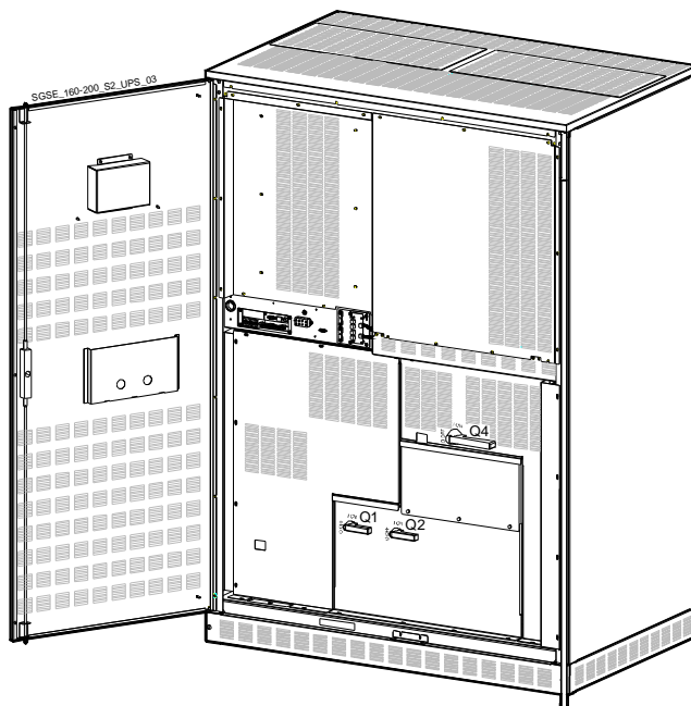
Рис. 2.1-2 Общий вид с открытой дверью
