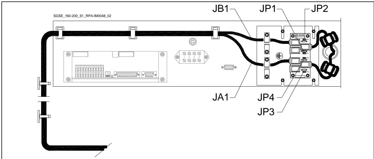
Рис. 5.9.2-2 Подключение кабеля на первом и последнем ИБП
