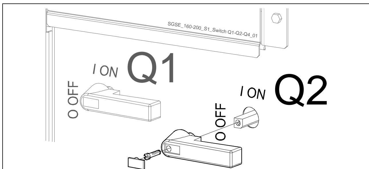
Рис. 5.8.6-1 Рубильник Q2 – Ручной Байпас
