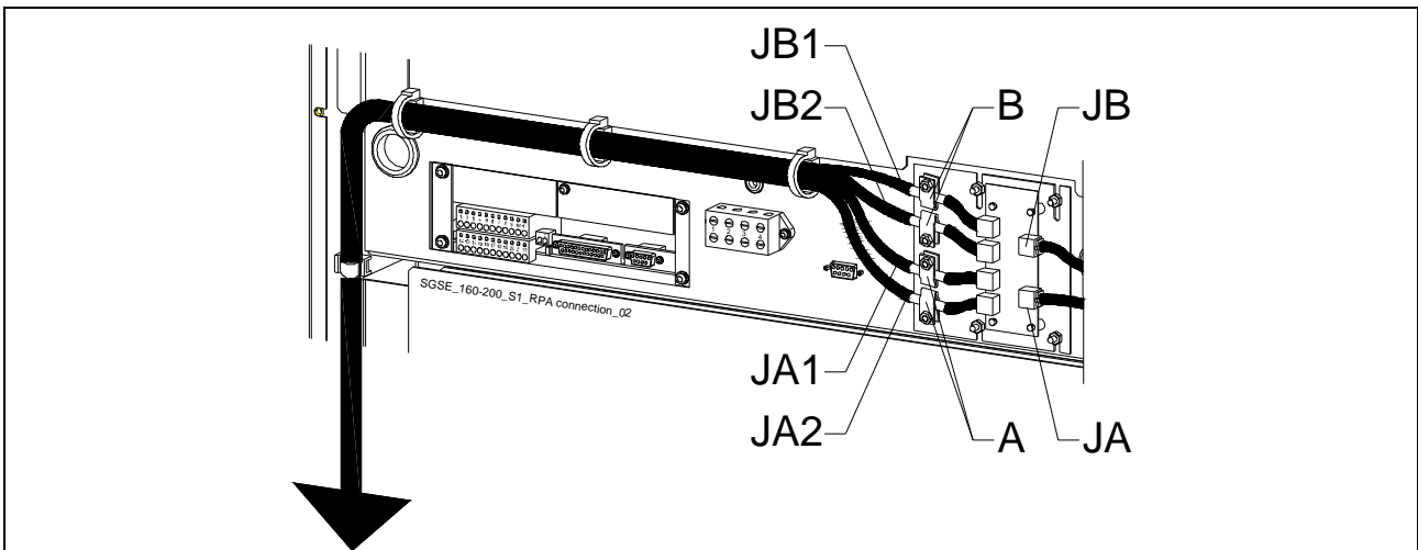
Рис. 5.9.3-2 Вид спереди на блок электроники промежуточных ИБП
