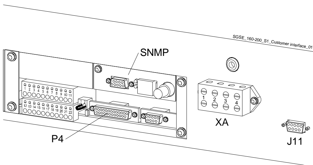
Рис. 2.1-5 Коммуникационный блок
